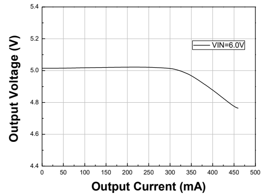
14. 输出电压VS带载
