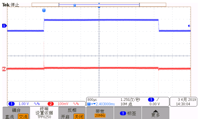
17. 输入电压瞬态响应(VIN=6.0~7.0V, IL=30mA)
